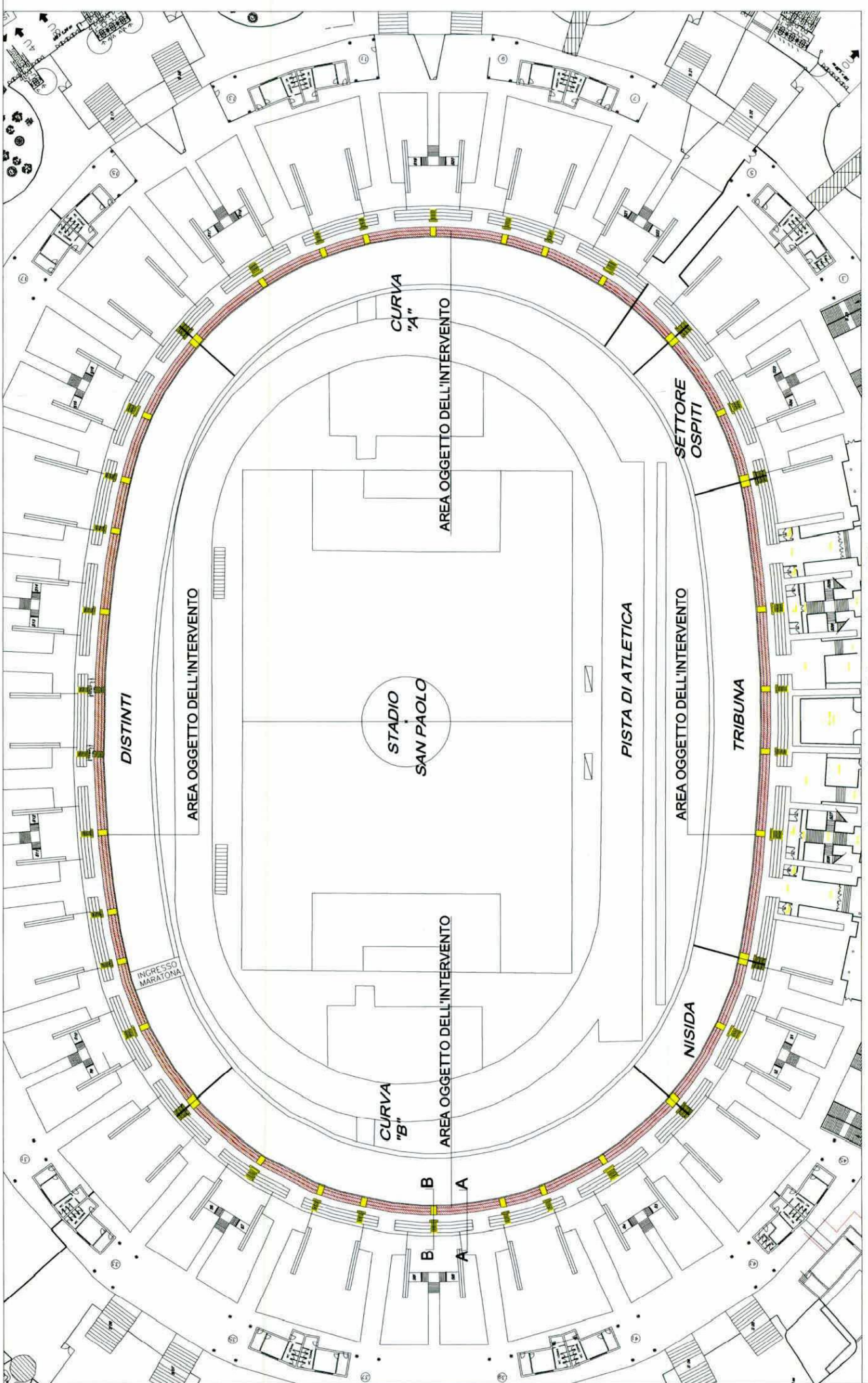
pianta anello superiore stato di fatto scala 1:500
